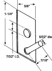
86-10 Pivot Pin
